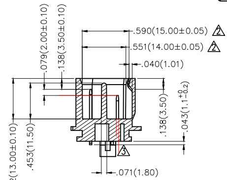
SEC A-A
