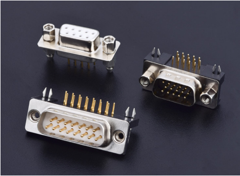
车针D-SUB连接器 Machined Terminal D-SUB Connectors
