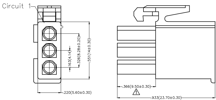
3 Circuits
