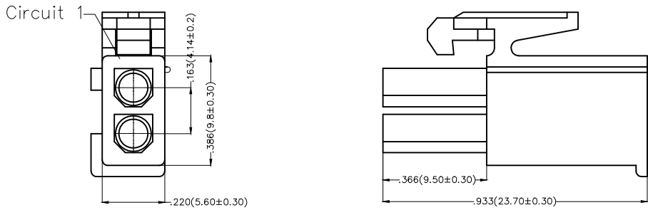
△ 2 Circuits
