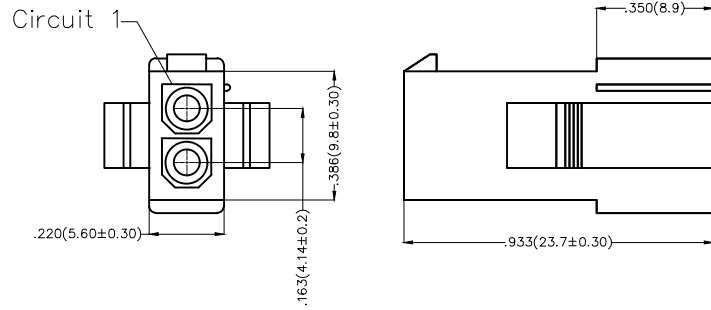
2 Circuits
