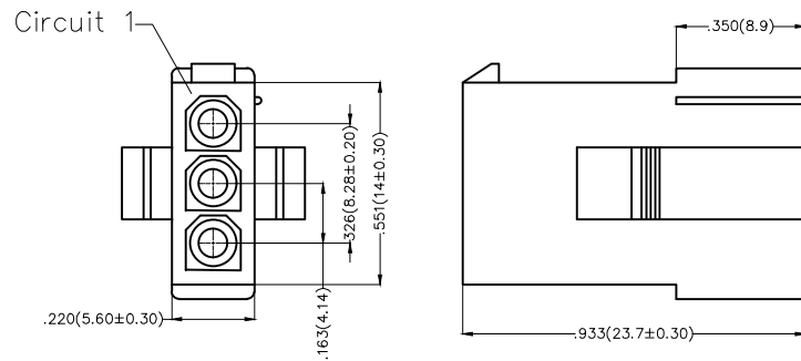
3 Circuits
